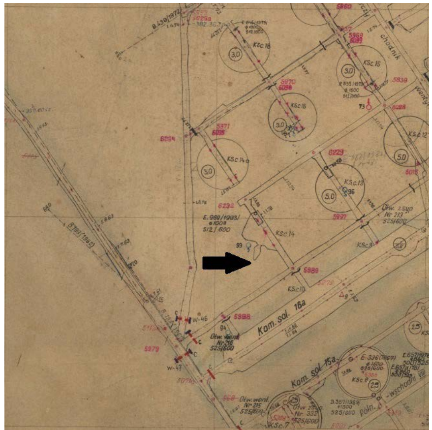
Rys. 4. Lokalizacja wycieku 93/525
